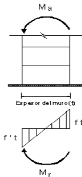
Figura 15: Momento Resistente en un muro de albañilería
