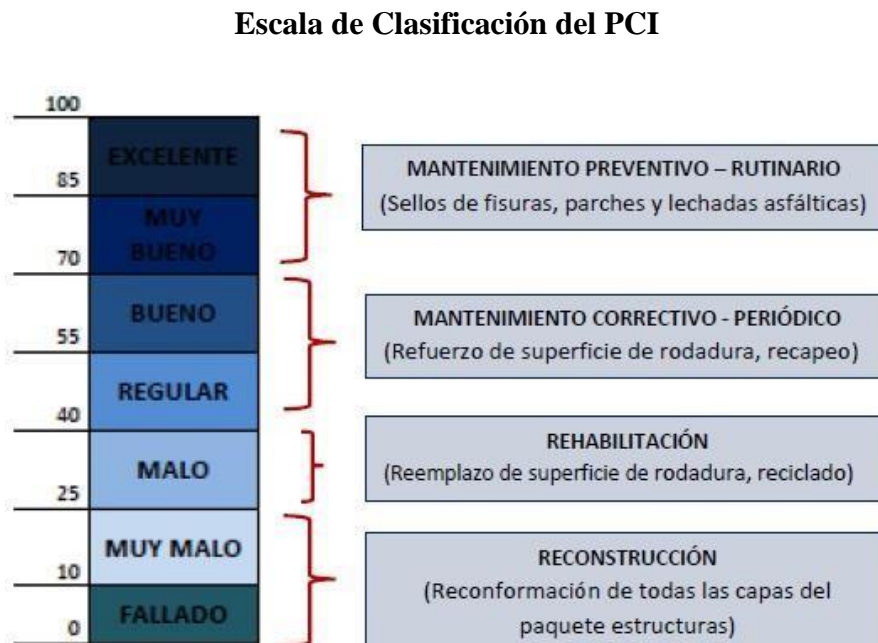
Figura 11 Escala de Graduación y tipo de intervención según escala de PCI.
