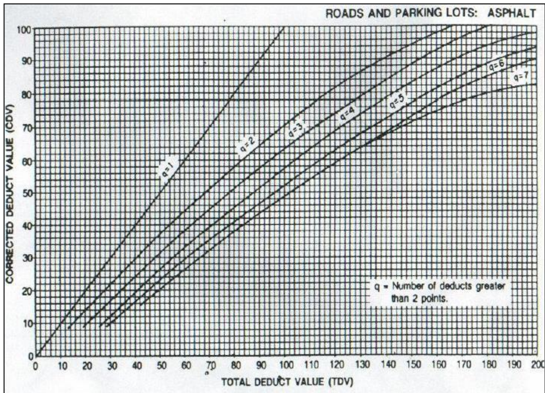
Figura 14. Curva de corrección para pavimentos
